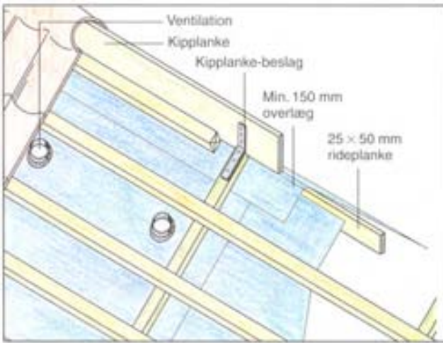
Figur 3. Kipløsning, hvor undertaget er ført op og fastholdt under kipplanken. Undertaget fastholdes mod kipplanke af lægte mellem spær. Løsningen kan også udføres uventileret ved at udføre undertaget med udluftningshætter.
