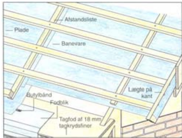
Figur 4. Ventileret foddetalje, hvor undertaget fastholdes til underlagsplade med fugebånd, så blafning undgås. Løsningen benyttes på samme måde, hvor der anvendes diffusionsåbne undertagsmaterialer, som ikke kræver ventilation i tagfladen.
